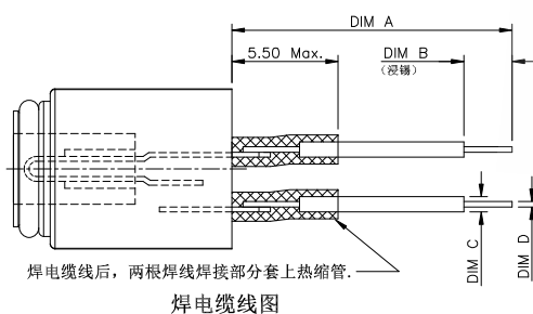
焊电缆线图
