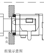
组装示意图
