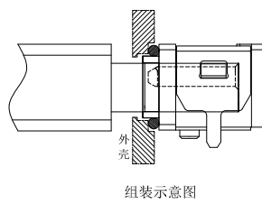
组装示意图
