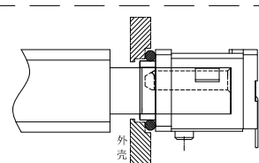
组装示意图
