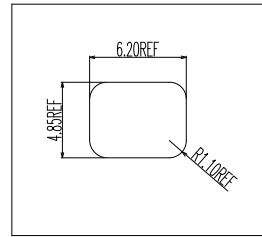
面板开孔参考尺寸
