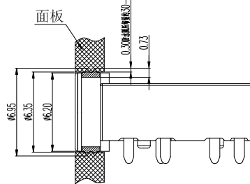
面板开孔建议尺寸 (ø6.35)
