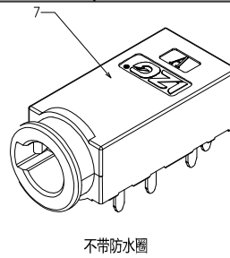
不带防水圈
